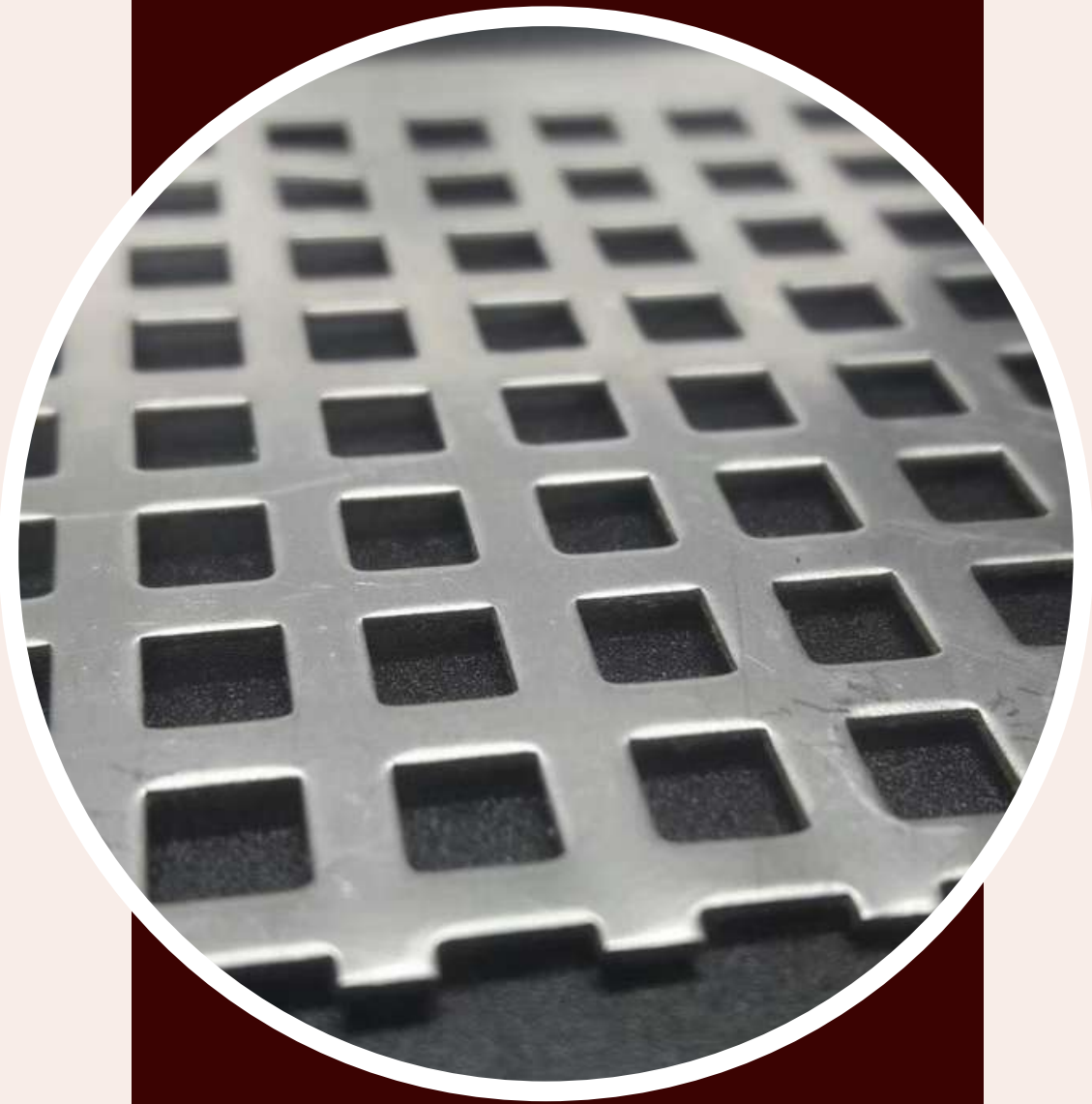
รูสี่เหลี่ยม 5x5 มม.
