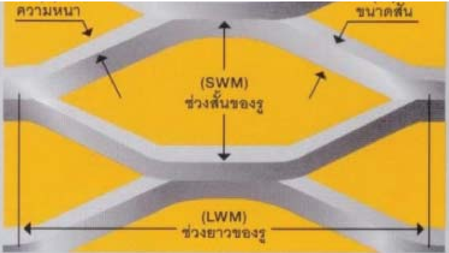
วิธีวัดขนาดรูกว้างxยาว เส้นตะแกรง และความหนาของตะแกรง
